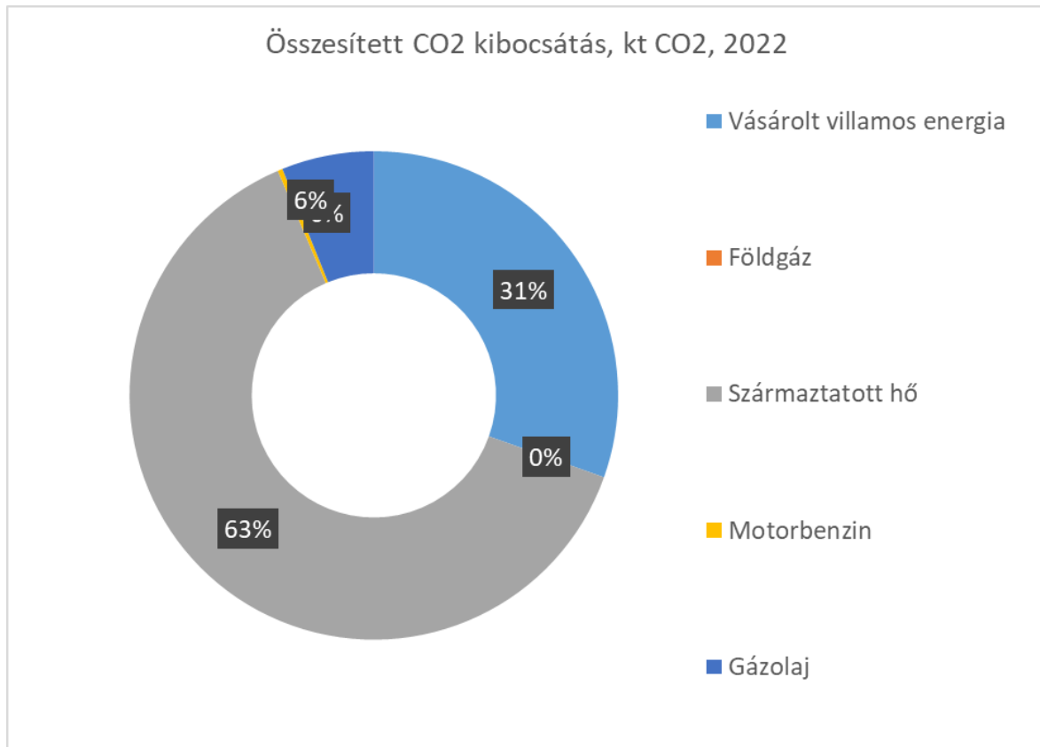
2. Ábra A Társaság összesített CO 2 kibocsátása energiahordozónként
