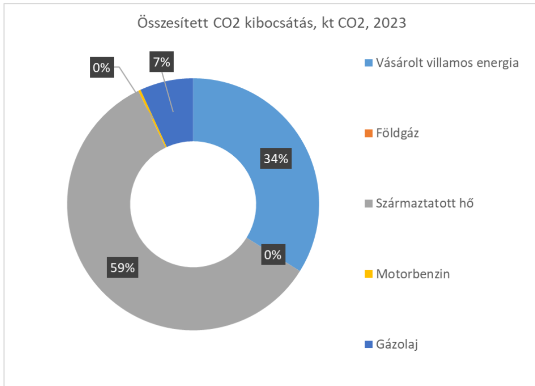
2. Ábra A Társaság összesített CO 2 kibocsátása energiahordozónként
