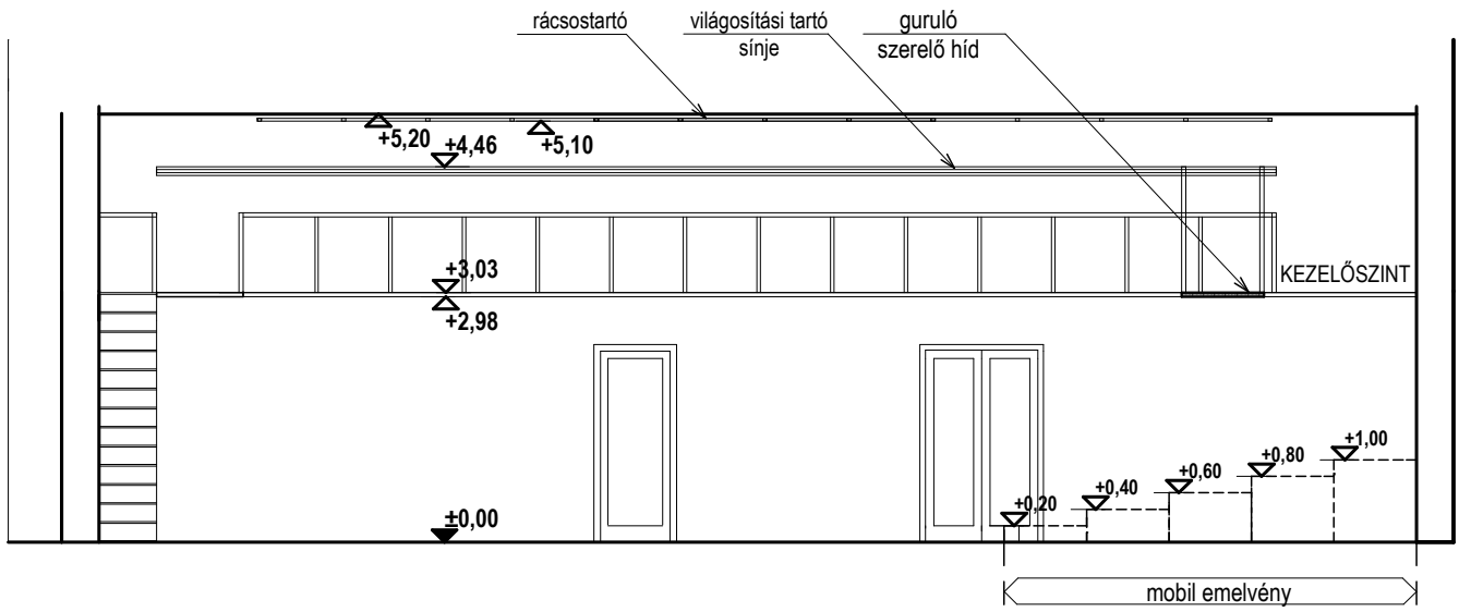
A-A METSZET
