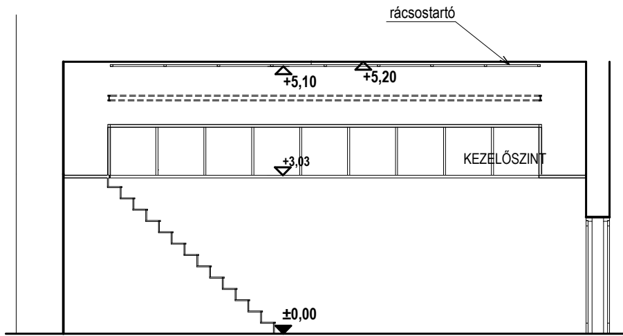
B-B METSZET
